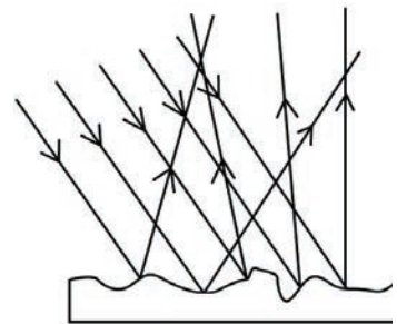
चित्र 7.24 अनियमित परावर्तन
