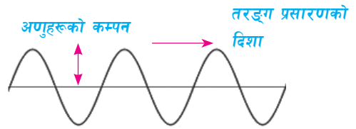
चित्र 7.16 ट्रान्सभर्स तरङ्ग
