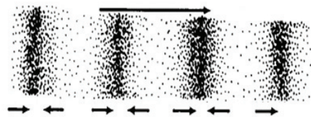
अणुहरूको कम्पन
